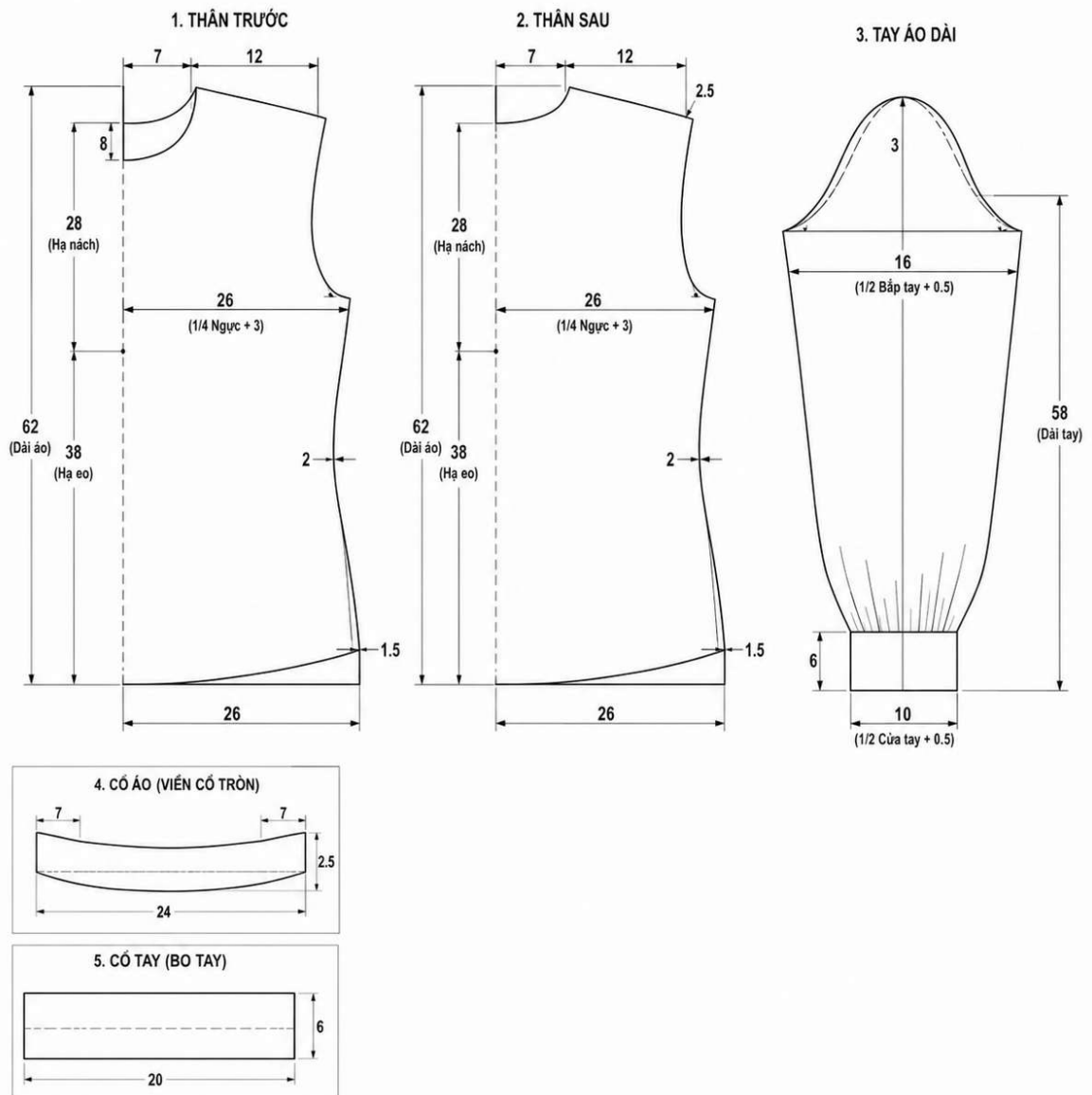
Hình 4: Ảnh mẫu rập sản phẩm mẫu
